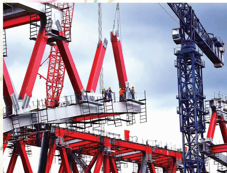
图片拍摄于延崇高速公路砖楼特大桥,因为工人正在进行钢梁吊装。李英军摄
